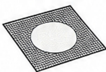
Wire Gauze
