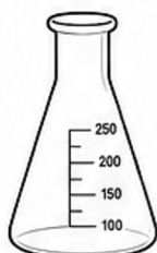
Erlenmeyer Flask
