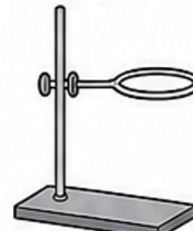
Ring Stand
